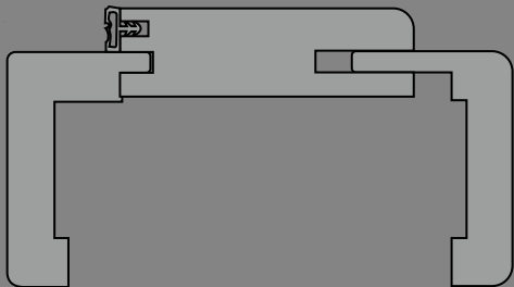
ZARGE MIT RUNDKANTE CHÂSSIS AVEC CHANTS ARRONDIS
